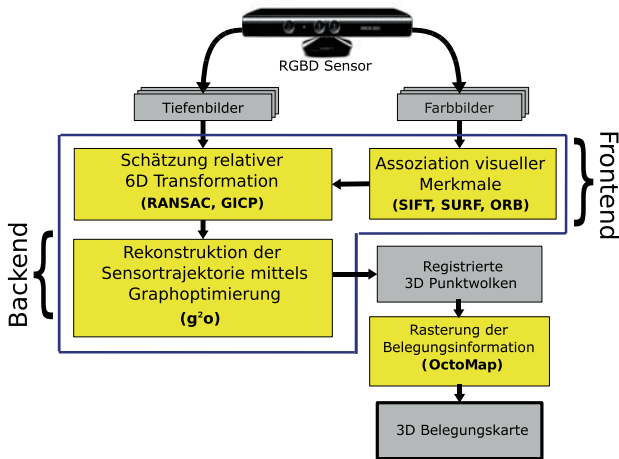
Bild 3 Überblick: Die Transformationen zwischen den Sensorposen einzelner RGB-D-Bilder werden über Merkmalsassoziationen oder Generalized Iterative Closest Point geschätzt. Aus den einzelnen Schätzungen wird durch Graphoptimierung die Trajektorie mit dem geringsten quadratischen Fehler berechnet. Diese ist die Grundlage zum Aufbau einer probabilistischen 3D-Belegungskarte aus den Sensordaten.
