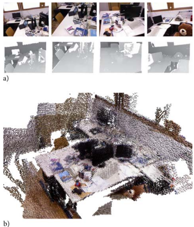
Bild 2 (a) Farb- und Tiefenbilder der Sequenz „FR1 Desk2“; (b) Resultierende 3D-Belegungskarte für „FR1 Desk2“.
