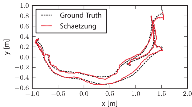
Bild 5 Die Rekonstruktion der Sensortrajektorie von Sequenz „FR1 Desk2“ im Vergleich zur Ground Truth des Bewegungserfassungssystems.
