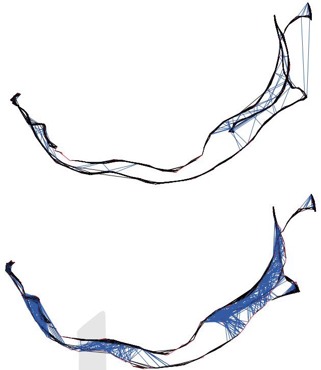
Bild 4 Posengraphen für die Sequenz „FR1 Desk2“. Blaue Kanten repräsentieren Loop Closures. Oben: Suche nach Transformation zu sequenziellen Vorgängern. Unten: Suche nach Transformation zu Nachbarn im Graph. Das Ausnutzen bestehender Loop Closures bewirkt eine deutlich stärkere Vernetzung des Graphen und somit auch eine Verminderung der Posensicherheit.
